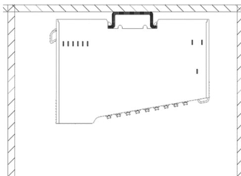
①垂直安装侧视图
