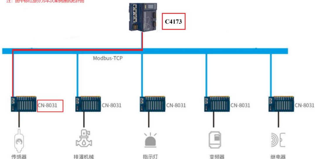
C4173 Modbus TCP客户端通讯拓扑图
