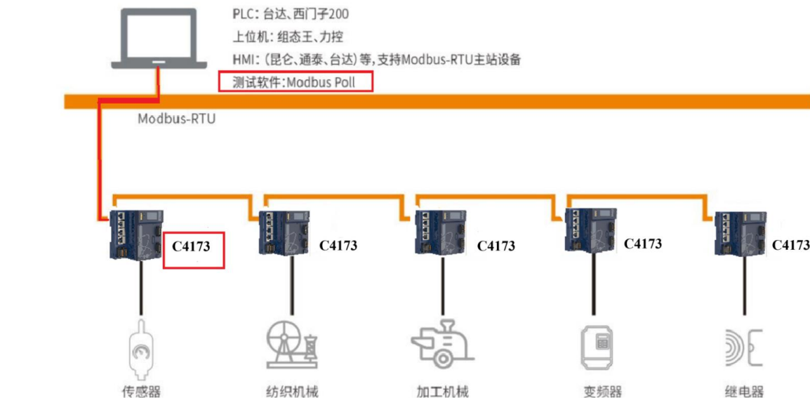
C4173 Modbus RTU从站通讯拓扑图
