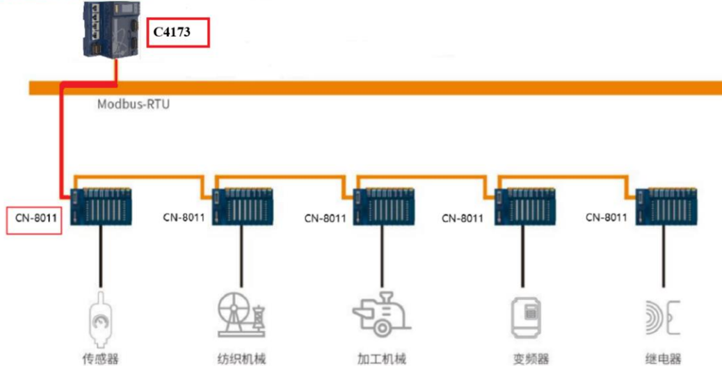
C4173 Modbus RTU主站通讯拓扑图
