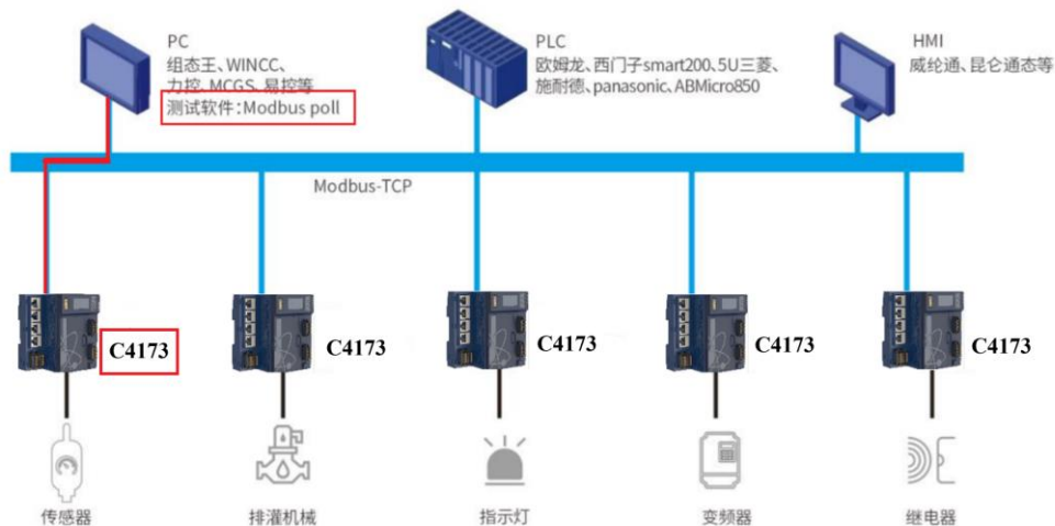
C4173 Modbus TCP服务器通讯拓扑图
